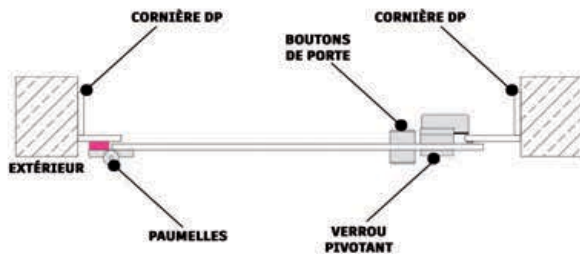
PORTE SUR TABLEAU MAÇONNÉ (ouv. extérieure) REZ/F21 à REZ/F24 (1800/1890mm) ou REZ/F31 à REZ/F34 (2000mm) Kit POIGNÉE PREMIUM ALU (ZZP82) ou INOX en option (ZZP83)
