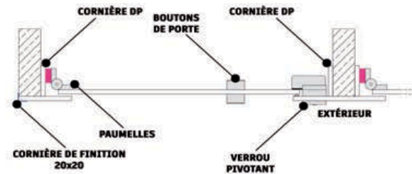
LES FAÇADES ET PORTES REZ/F41 à REZ/F56 (1855 / 2000mm) Kit IMPOSTE 150mm en option (ZZP09)
