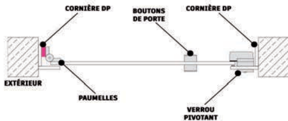
PORTE SUR TABLEAU MAÇONNÉ (ouv. intérieure) REZ/F21 à REZ/F24 (1800/1890mm) ou REZ/F31 à REZ/F34 (2000mm) Kit PORTE COULISSANTE en option (ZZP07)
